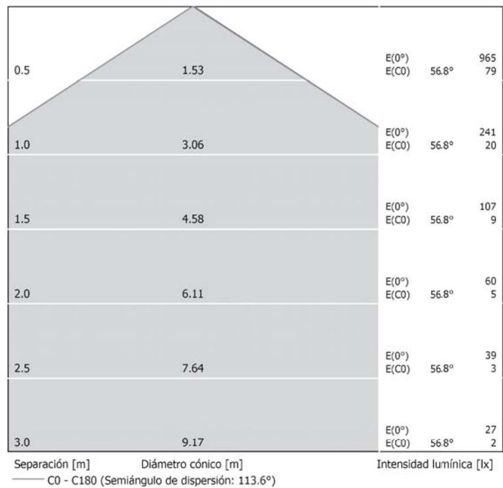
Diagrama Cónico
