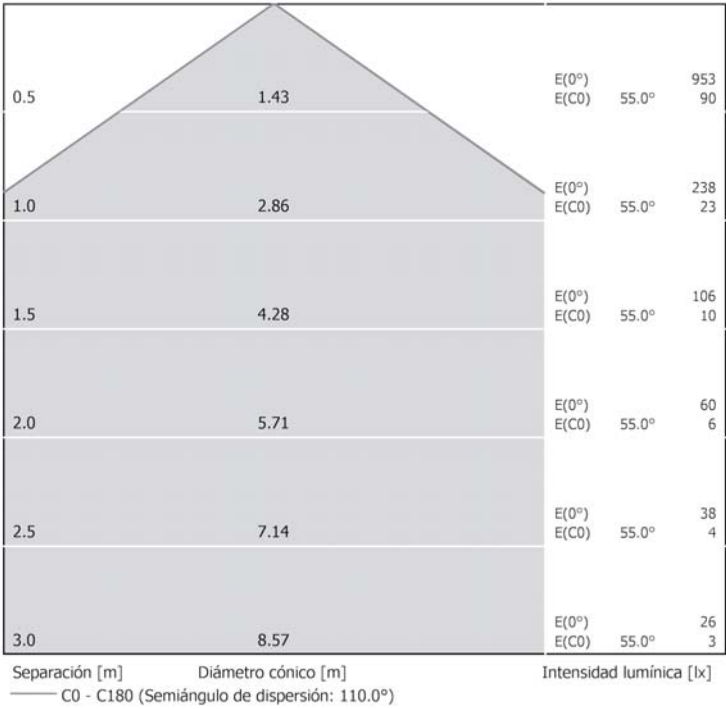
Diagrama Cónico
